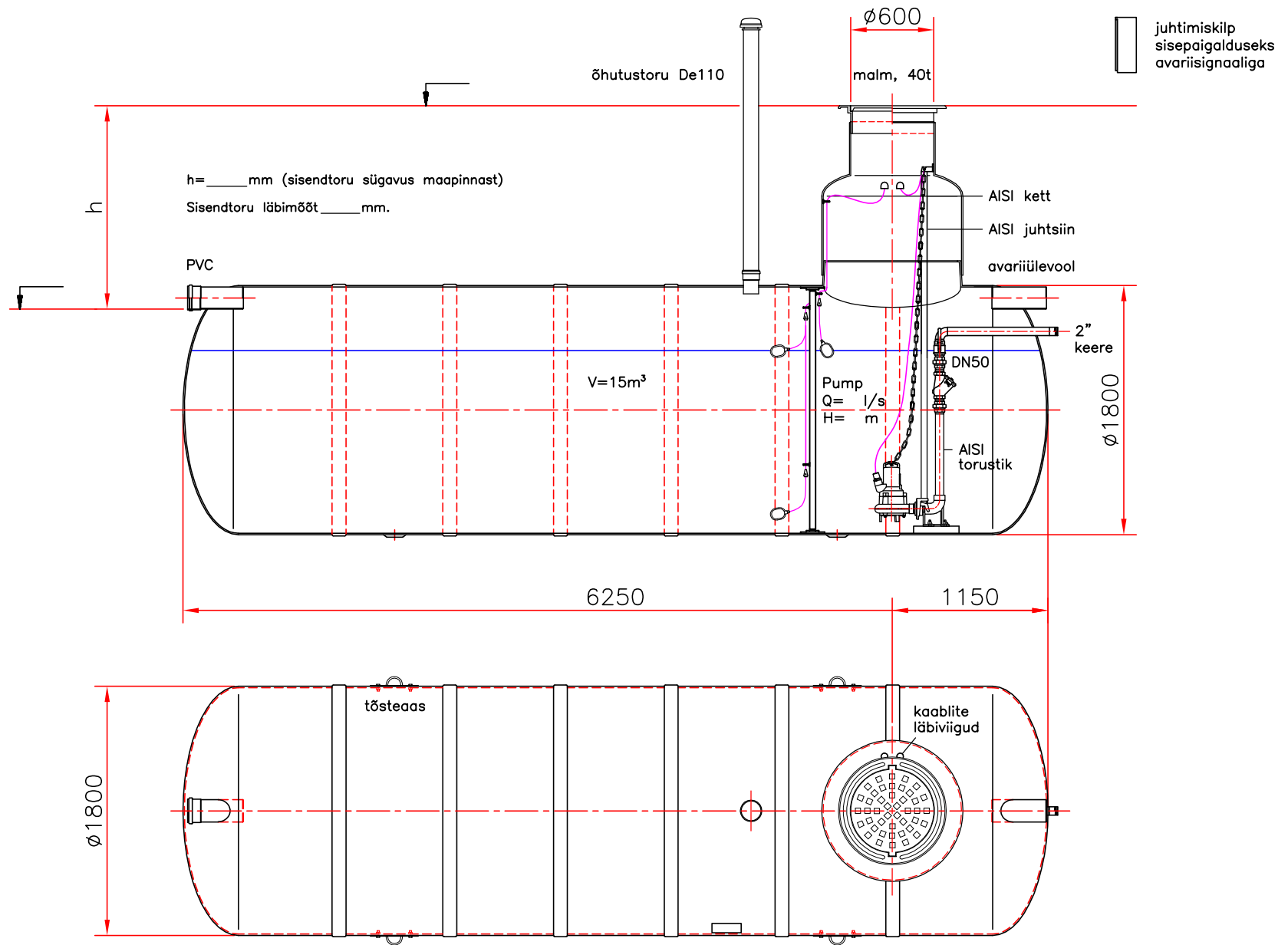
Joonise nimetus: 15 M 3 SADEMEVEE ÜHTLUSTUSMAHUTI-PUMPLA
